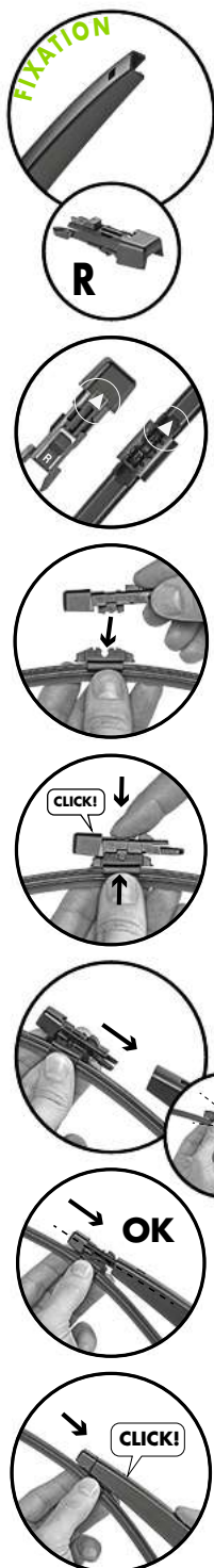
Fitting Instruction de montage N° 1R
